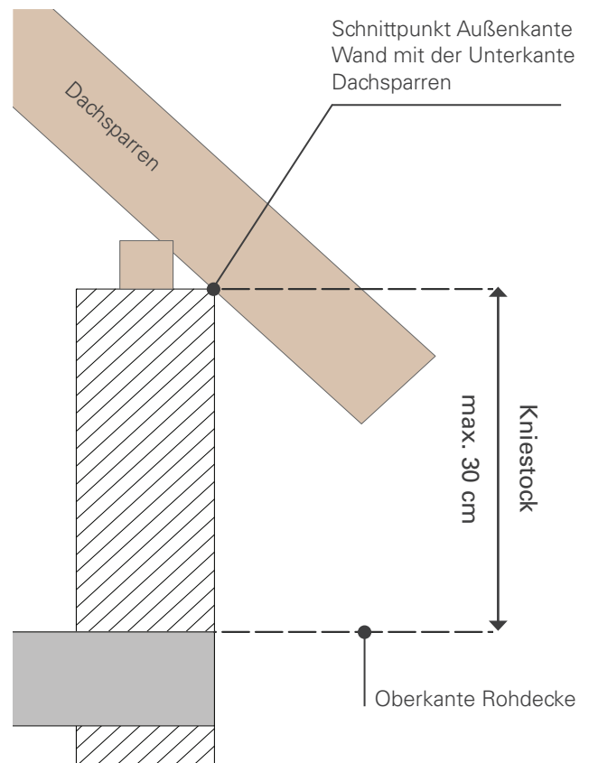
Zeichnerische Begriffserläuterung zum Kniestock
